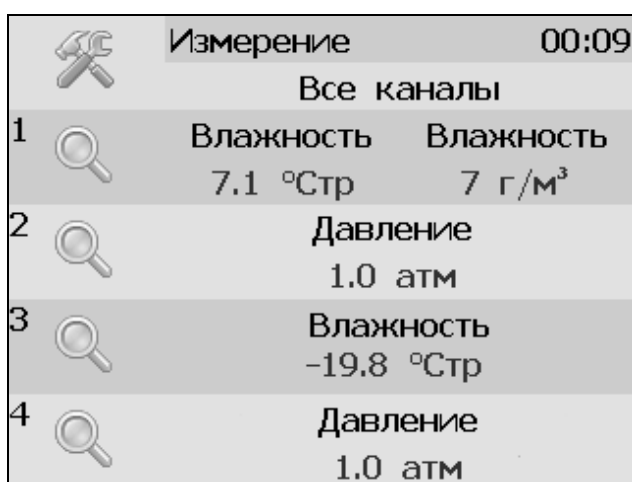
Рисунок 3.2 Вид главного экрана каналов измерений: а) ИВГ-1 /1-Т-4Р-2А(-Е); б) ИВГ-1 /2-Т-4Р-2А(-Е);
