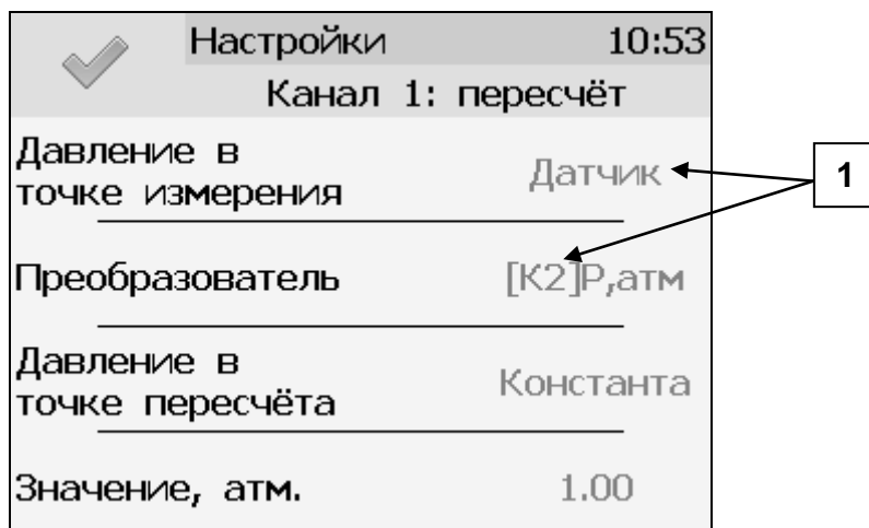
Рисунок 6.13 Настройка параметров пересчета влажности
