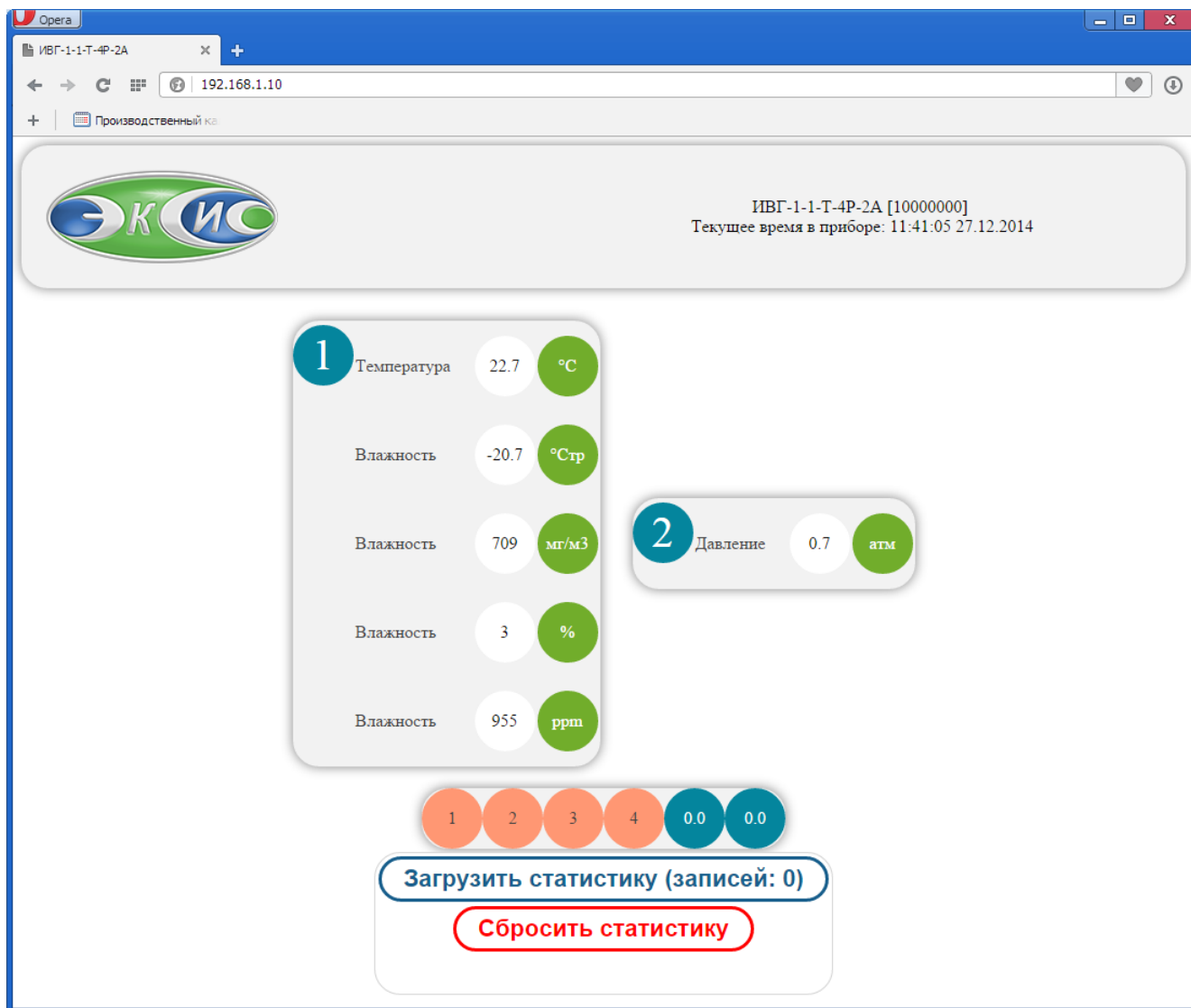
Рисунок 6.32 Web-интерфейс прибора ИВГ-1 /1-Т-4Р-2А-Е.
