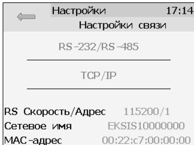
Рисунок 6.27 Экран настроек связи (ИВГ-1 /Х-Т-4Р-2А-Е)
