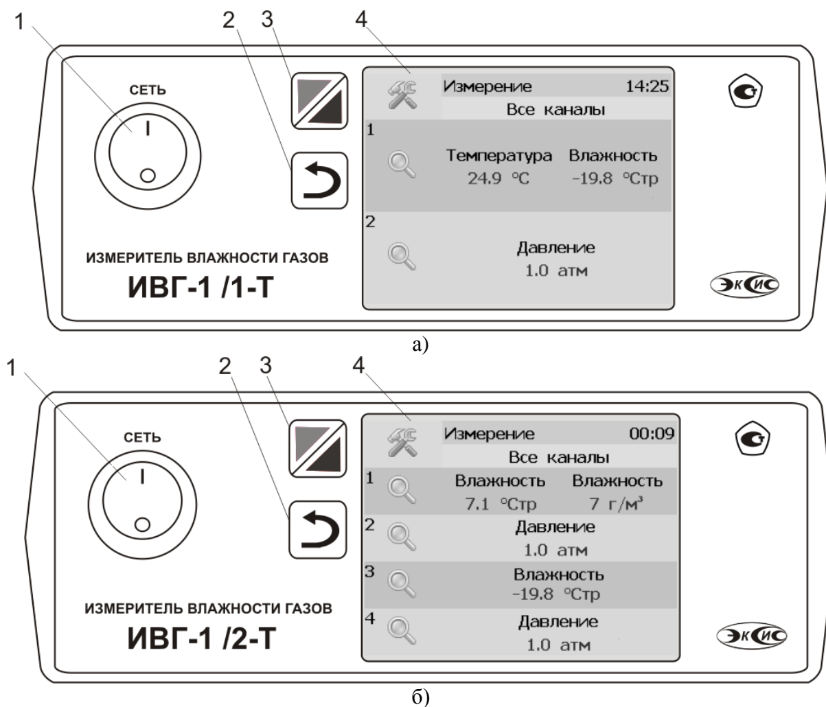
Рисунок 3.1 Вид лицевой панели измерителя: а – одноканального исполнения б - двухканального исполнения
