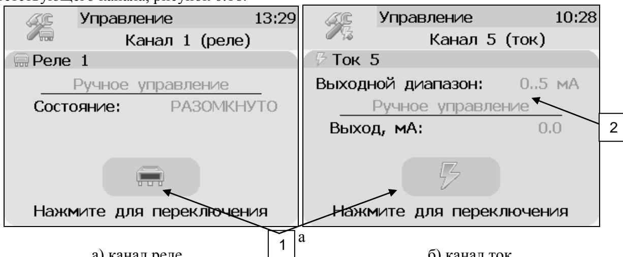
а) канал реле б) канал ток Рисунок 6.11 Виды экрана первого и пятого канала управления
