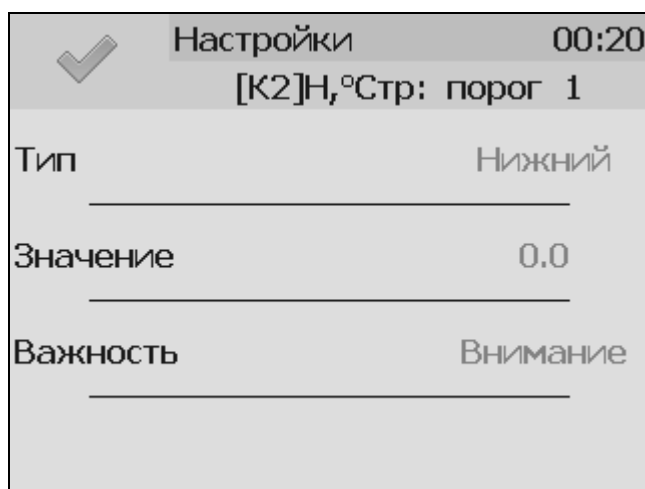
Рисунок 6.6 Экран настройки второго порога для абсолютной влажности (Ст.р.).
