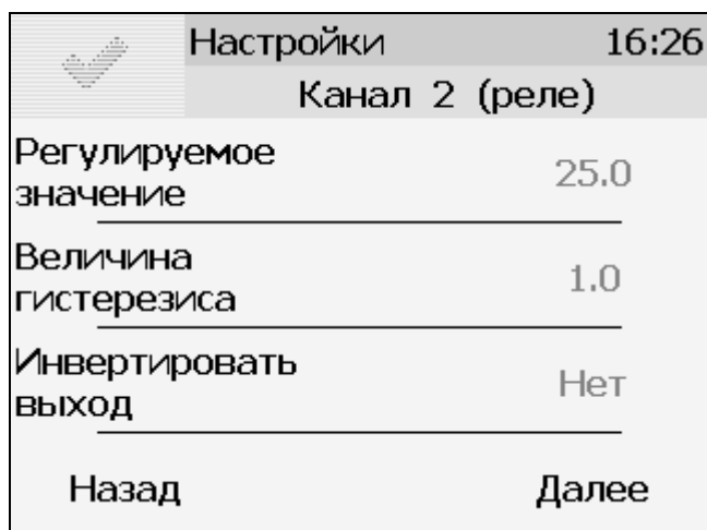
Рисунок 6.19 Вид экрана настройки гистерезис
