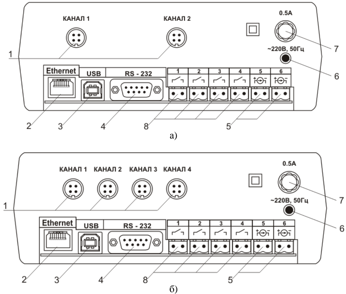
Рисунок 3.4 Вид задних панелей приборов ИВГ-1 /X-T-4P-2A-E (3): а - одноканального исполнения б - двухканального исполнения
