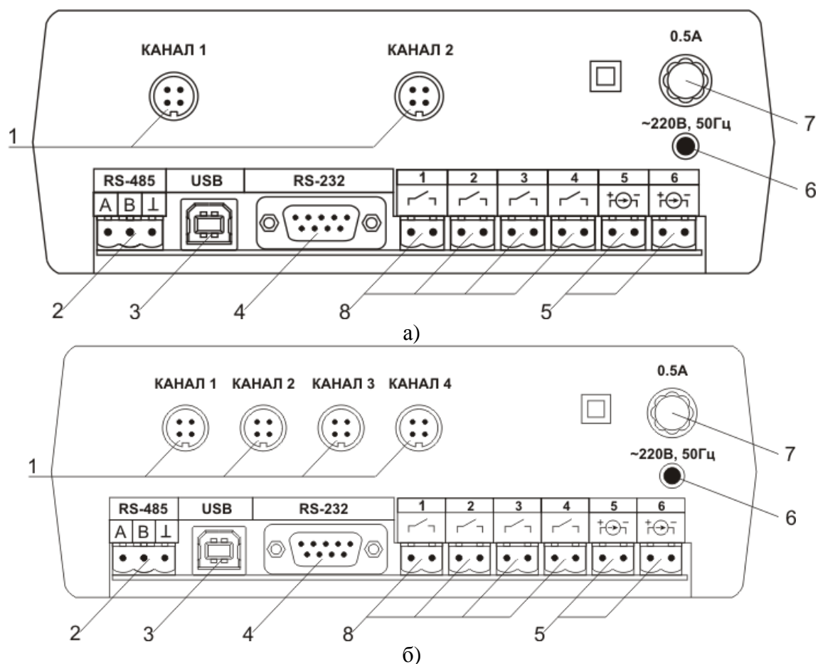
Рисунок 3.3 Вид задних панелей приборов ИВГ-1 /X-T-4P-2A (3):
