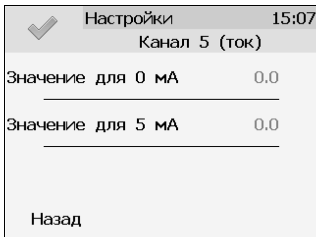
Рисунок 6.25 Вид экрана настройки линейного токового выхода 0...5 мА.
