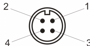
Рисунок 3.4 Разъем подключения преобразователей 1 – сигнал "А" линии RS-485 2 – сигнал "В" линии RS-485 3 – общий провод 4 – питание +12 В
