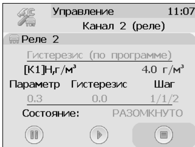
Рисунок 6.23 Экран канала управления с настроенной программой.
